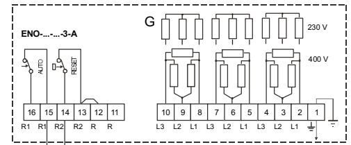
trzy sekcje grzewcze
