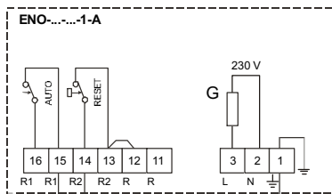
jedna sekcja grzewcza
